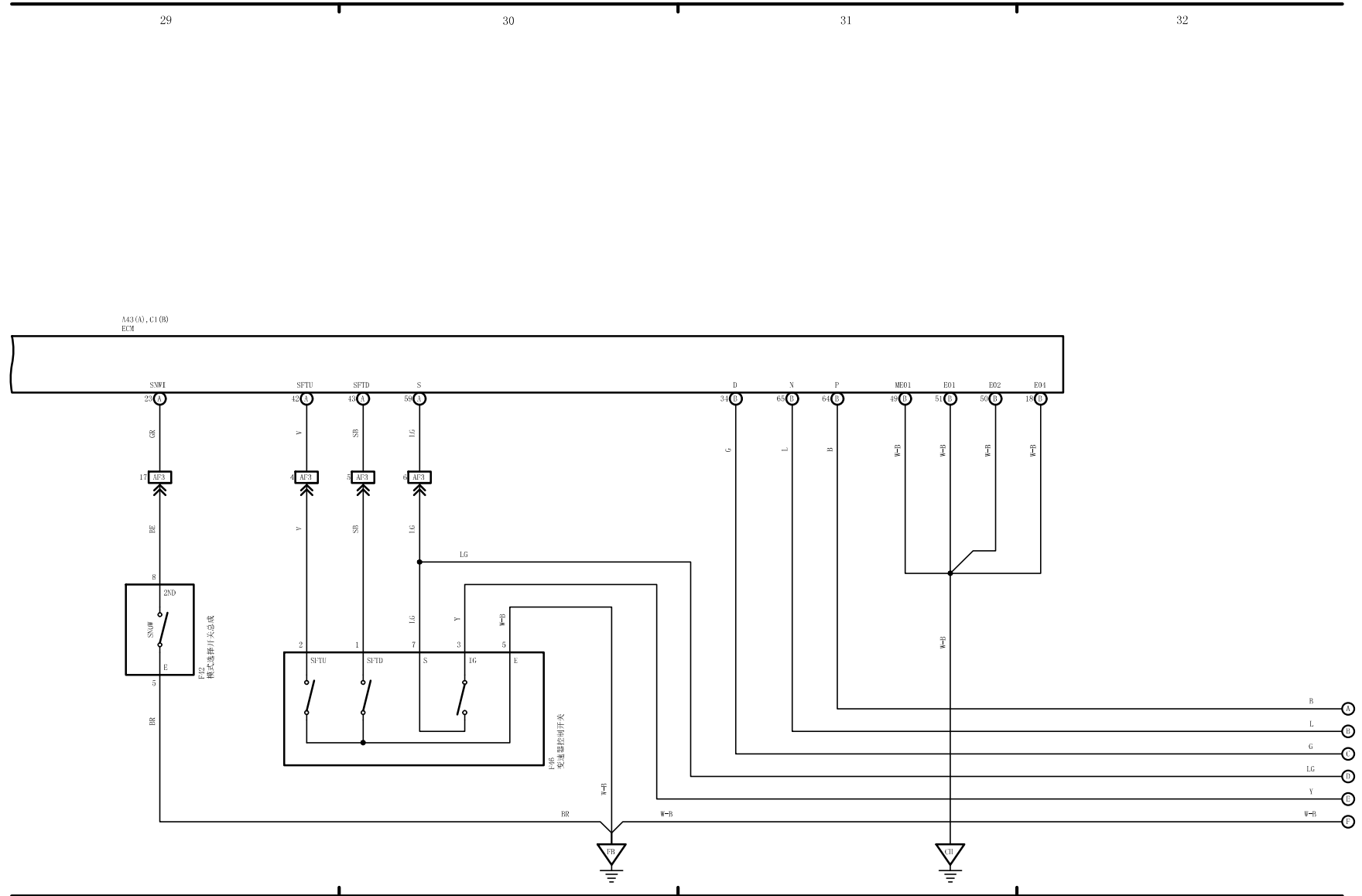
ECT 和 A/T 指示灯 (8AR-FTS)
