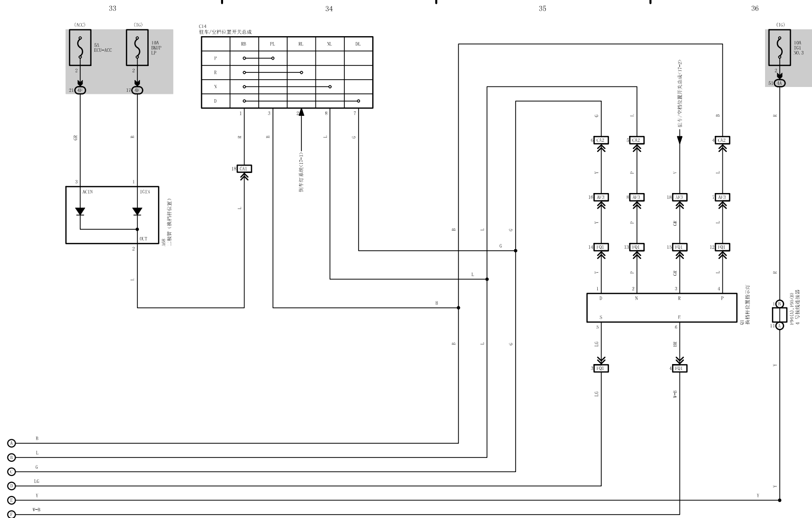
ECT 和 A/T 指示灯 (8AR-FTS)
