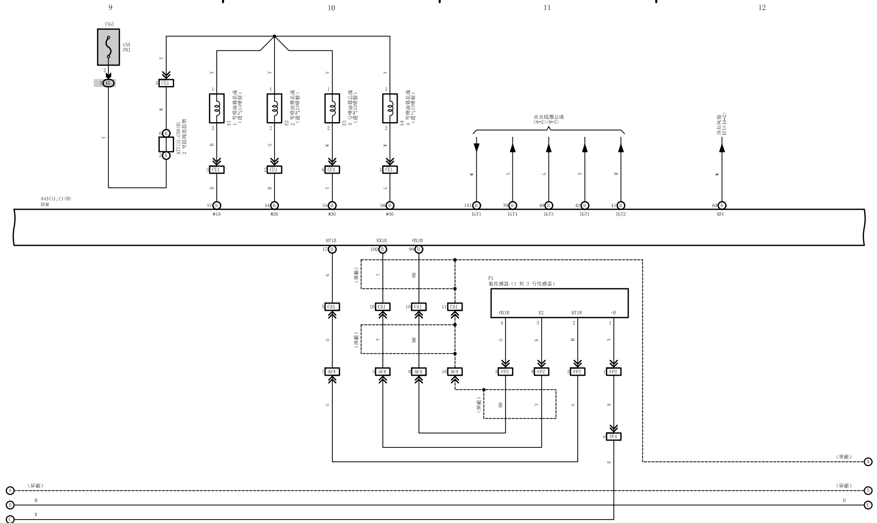
发动机控制 (8AR-FTS)
